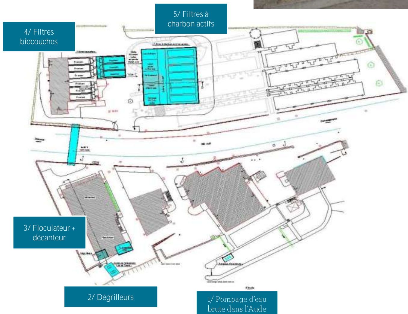
Figure 6 : schéma de l'usine de traitement de l'eau potable de Maquens
