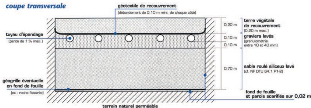
coupe transversale
